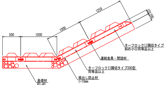
標準断面図 S=1:3
