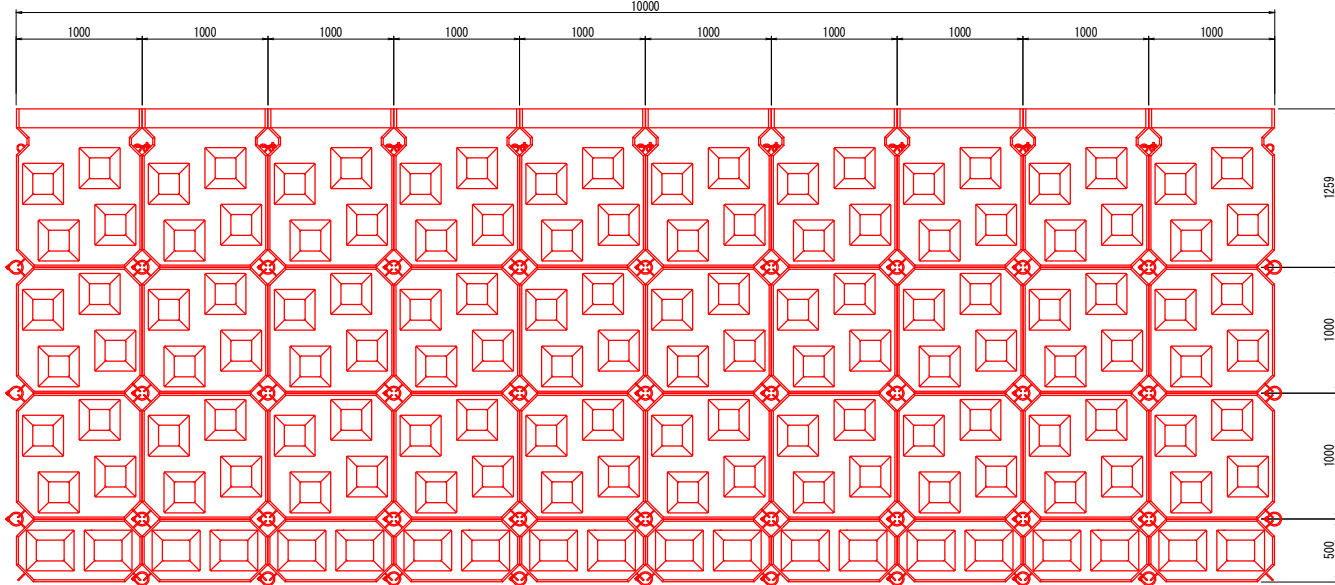
平場ブロック形式割付図 S=1:30
