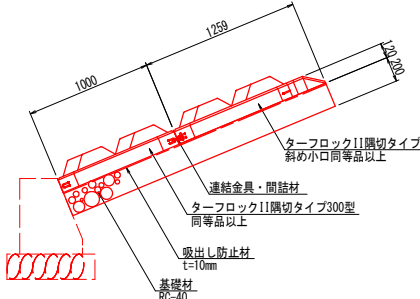
標準断面図 S=1.3
