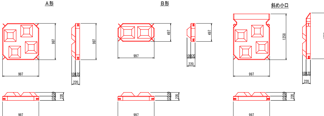
ブロック規格図
